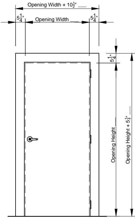
① SCALE: 3/8" = 1'-0"
