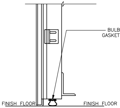
⑬ SCALE: 1" = 1'-0"
