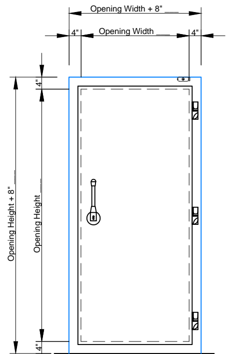
⑤ SCALE: 3/8" = 1'-0"
