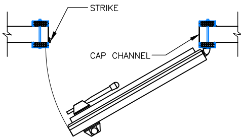
⑮ SCALE: 1/2" = 1'-0"
